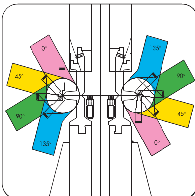
DIMEFORM® positive/negative Biegung : 0/135°
