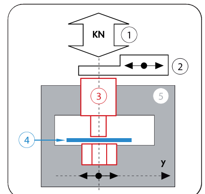
Die Multi-Step- Technologie
