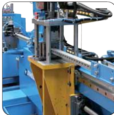
Mitlaufende Schere
