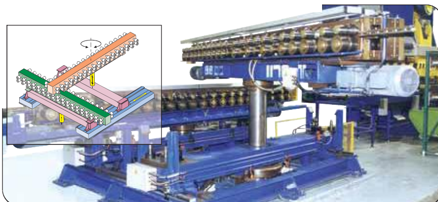
Profilieranlage mit drehbarer Schnellwechselkassette
