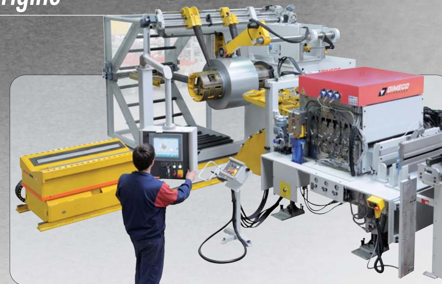
Alimentation de presse "Ligne courte"
