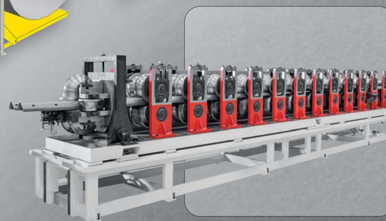
Profileuse et galets de profilage
